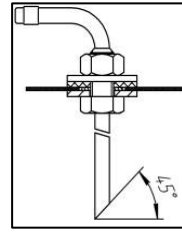
Abb. 15a - Installation des Kraftstoffsaugschlauches
