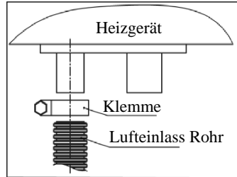
Fig. 4 – Anschluss der Luftleitung an das Heizgerät
