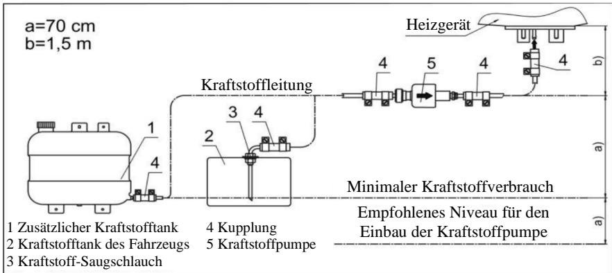
Abb. 19 – Höhenposition der Kraftstoffpumpe im Kraftstoffsystem
