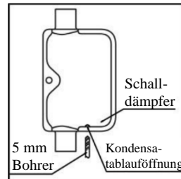
Abb. 10b – Kondensatablaufbohrung für vertikale Montage
