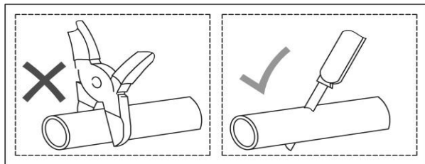
Abb. 21 - Schneiden der Leitung vor der Installation
