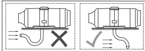
Fig. 5 – Position des Luftansaug-/Abgasrohrs
