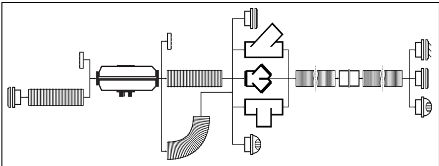
Abb. 26a - Luftkanalanschlüsse für AIR-2D (60mm)
