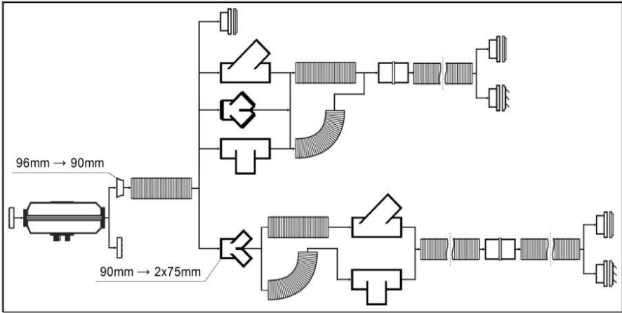
Abb. 26b - Luftkanalanschlüsse für AIR-4D (90mm/75mm)
