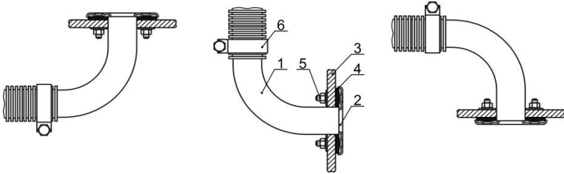
Abb. 7 - Montage des Luftansaugrohres
