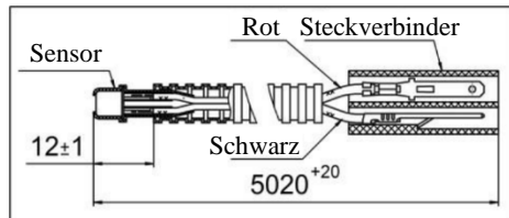
Abb. 23 - Temperatursensor
