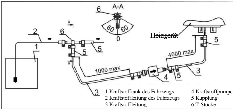
Abb. 17 - Kraftstoff Ansaugung mit einem T-Stück
