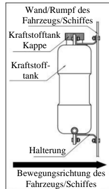
Abb. 16 Installation des Kraftstofftanks
