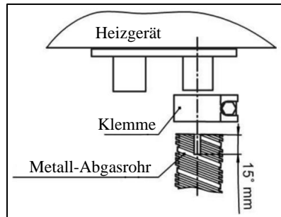
Abb. 8 - Befestigung des Metallrohres am Heizgerät
