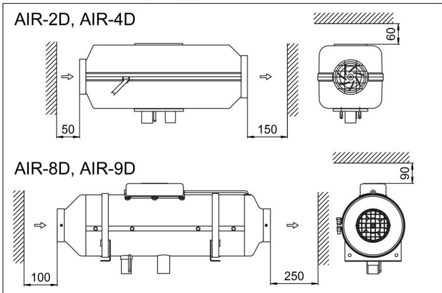
Abb. 1b –Abstand zu den Wänden
