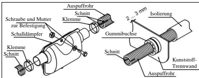
Abb. 11 - Befestigung des Auspuffrohres am Heizgerät und Verwendung von Gummibuchsen
