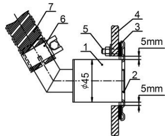
Abb. 13 - Montage des Auspuffrohrs
