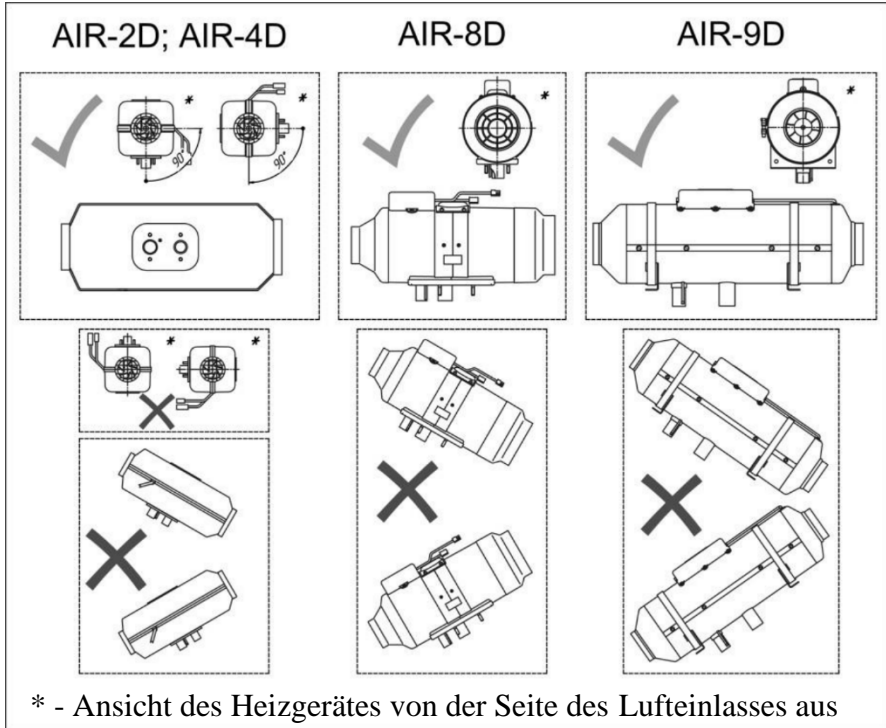
Abb. 1a - Einbaulagen des Heizgerätes
