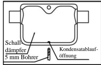
Abb. 10a - Kondensatablaufbohrung für horizontale Montage
