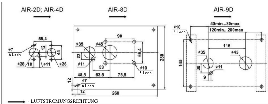
Abb. 3 – Befestigungsbohrungen
