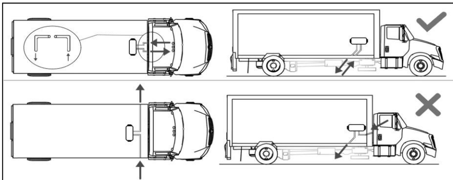
Abb. 6a - Lage der Ein- und Auslassleitungen an Landfahrzeugen
