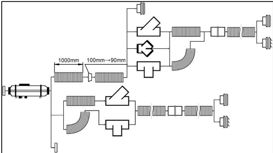
Abb. 26c - Luftkanalanschlüsse für AIR- 9D (100mm/90mm)
