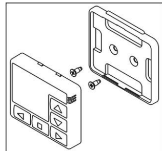
Abb. 24 – Montage des Bedienfeldes PU-27 mit einer Montagehalterung
