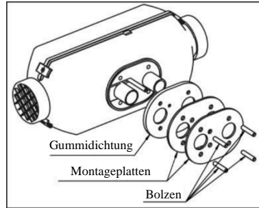
Abb. 2a - Montageplatten
