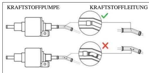
Abb. 21a - Anschlüsse der Kraftstoffleitung
