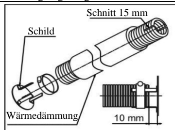
Abb. 9 - Auspuffrohrschild
