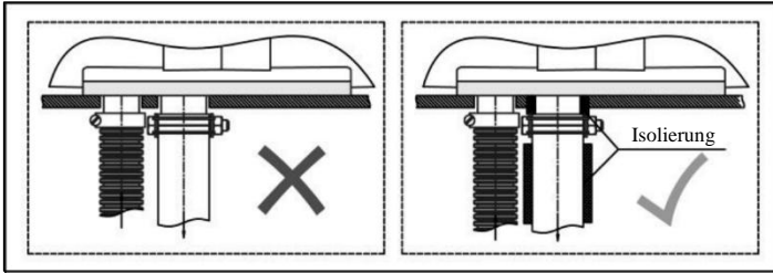
Abb. 12 - Einbau einer zusätzlichen Wärmedämmung
