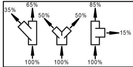
Abb. 25 - Beispiele für die Luftverteilung mit verschiedenen Komponenten
