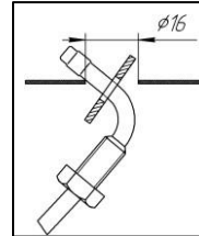
Abb. 15b - Installation der Unterlegscheibe
