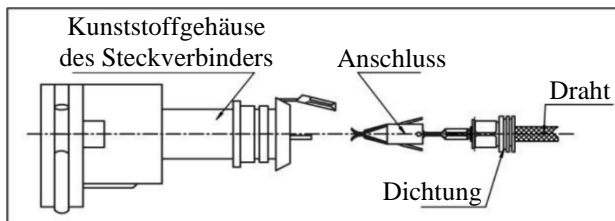
Abb. 22 - Installation des Anschlusses des elektrischen Kabelbaums der Kraftstoffpumpe
